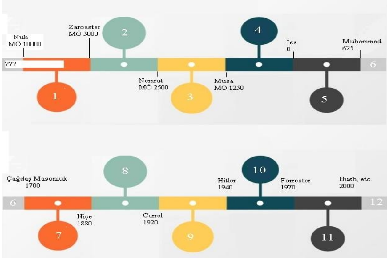
Şekil 2: Nesnel olarak seçilmiş kilit olaylar.
