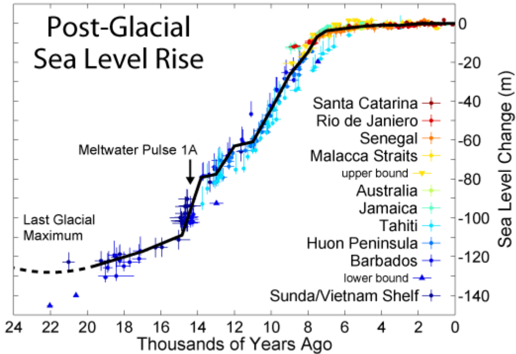
Şekil 5: Son buzul erimesinin zamana bağlılığı.
