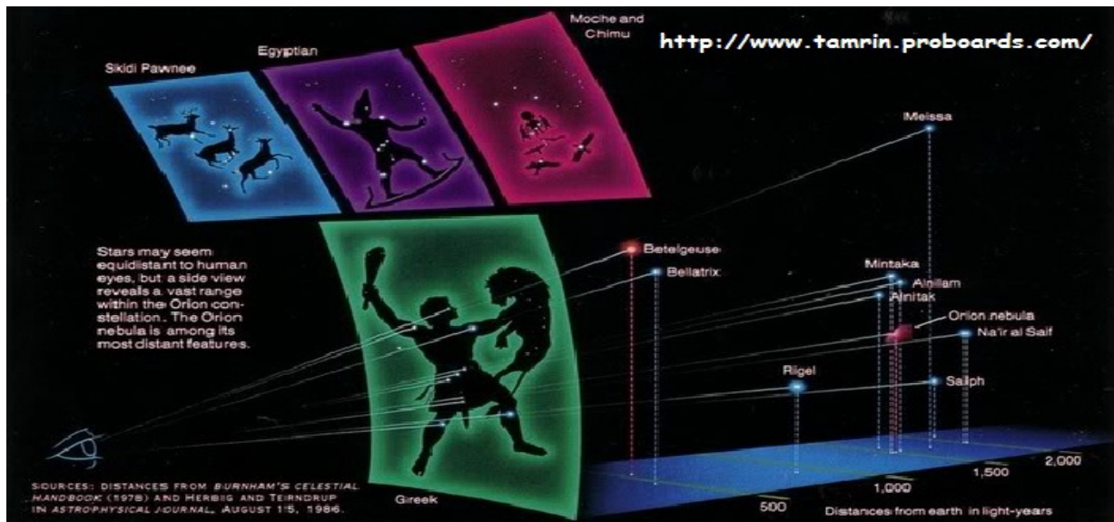
Şekil 17: Orion ile Dünya arasında mesafeler. Bu mesafelerde değişik kaynaklar arasında tam uyuma yok, be nedenle en az değişik 2-3 kaynaktan öğrenmek ve değerlendirmek gerekmektedir.
