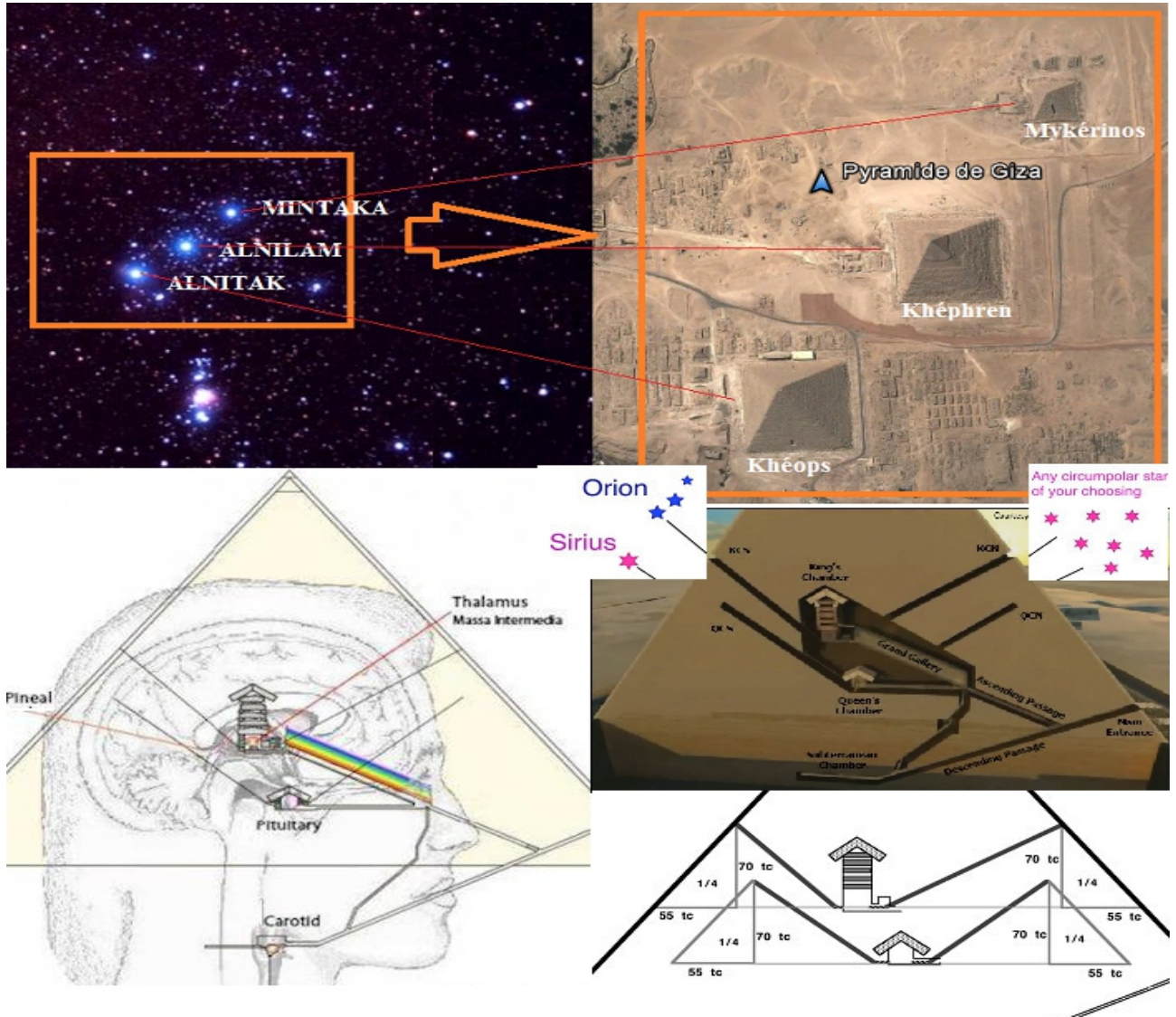
Şekil 19: Orion Gizemi ve Büyük Piramit.
